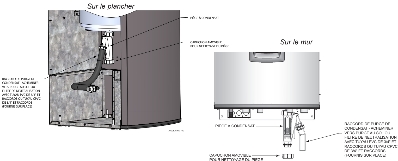
Figure 2-2 Rejet du condensat
